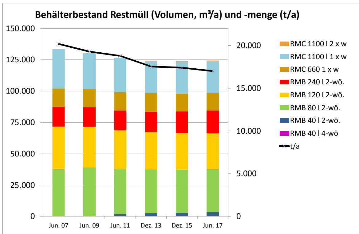
Abbildung 3: Restabfall Behältervolumen (m³/a) und Menge (t/a)
